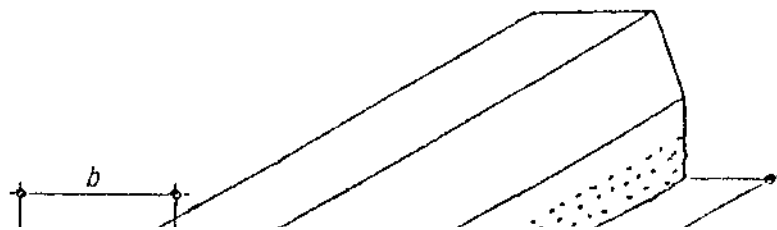
Rys. 3. Krawężnik mostowy rodzaju A
